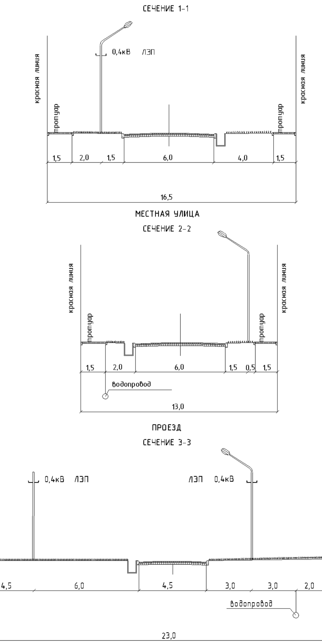
ПОПЕРЕЧНЫЕ ПРОФИЛИ МЕСТНОЙ УЛИЦЫ
