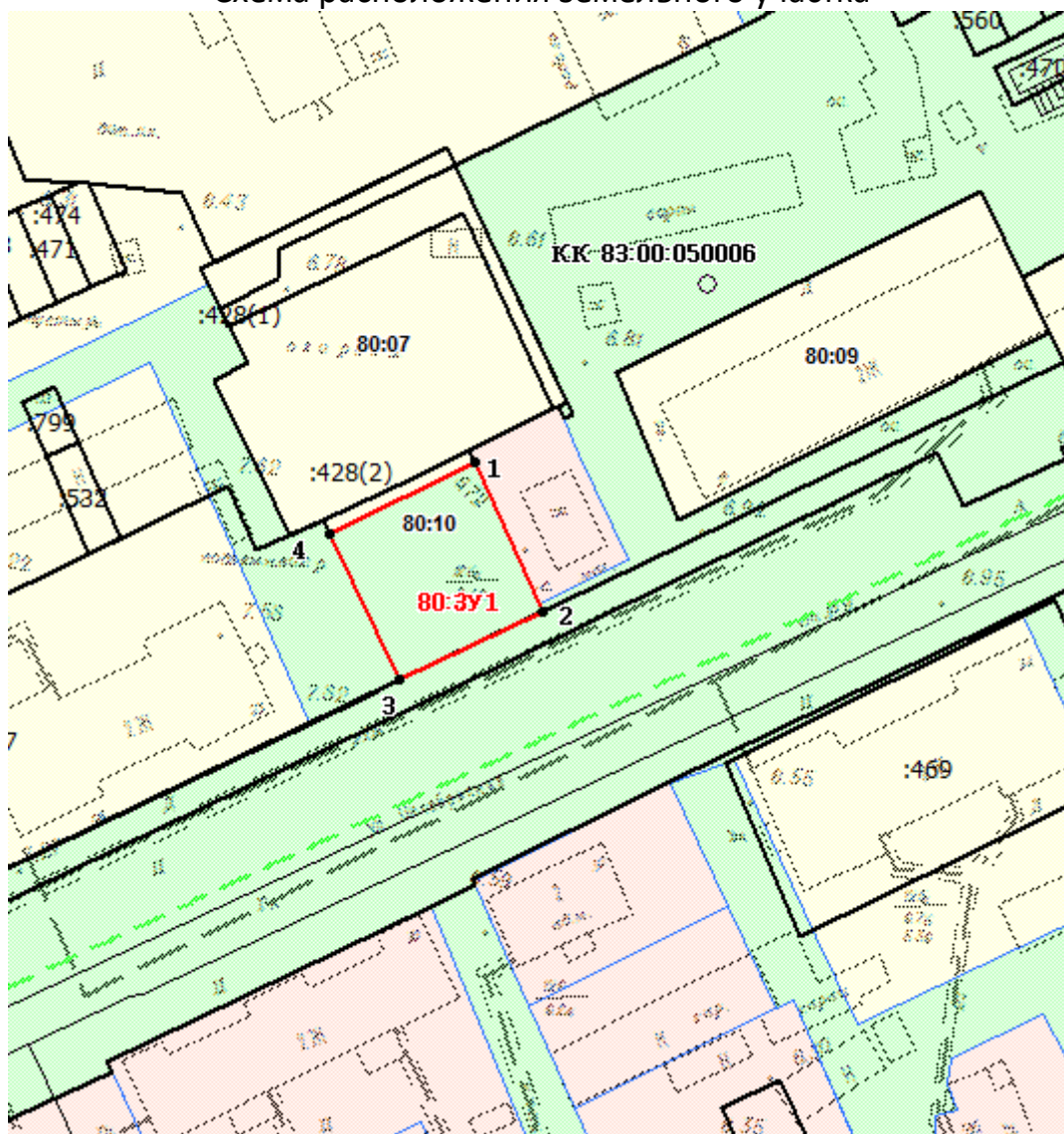
Схема расположения земельного участка
